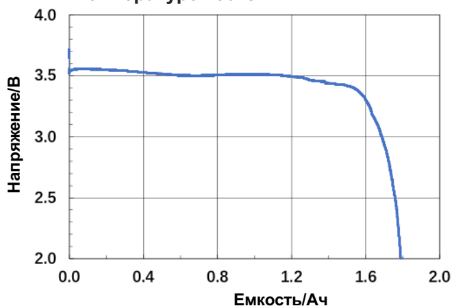
График разряда током 50 мА при температуре 150°C
