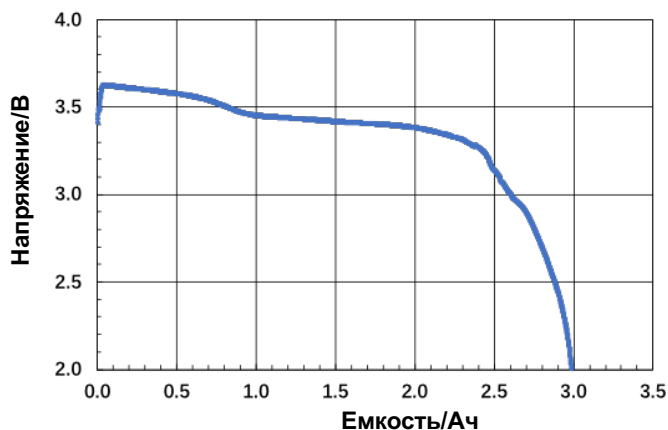
График разряда током 75 мА при температуре 165°C
