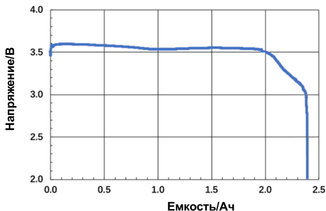
График разряда током 50 мА при температуре 165°C
