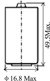
Размер (мм)
