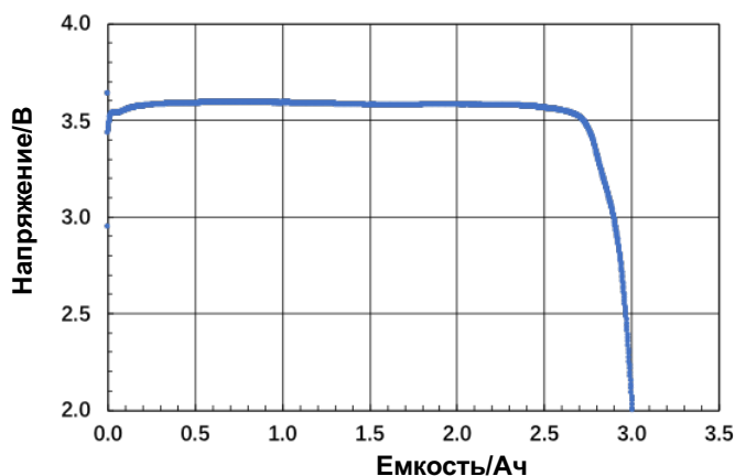
График разряда током 50 мА при температуре 150°C
