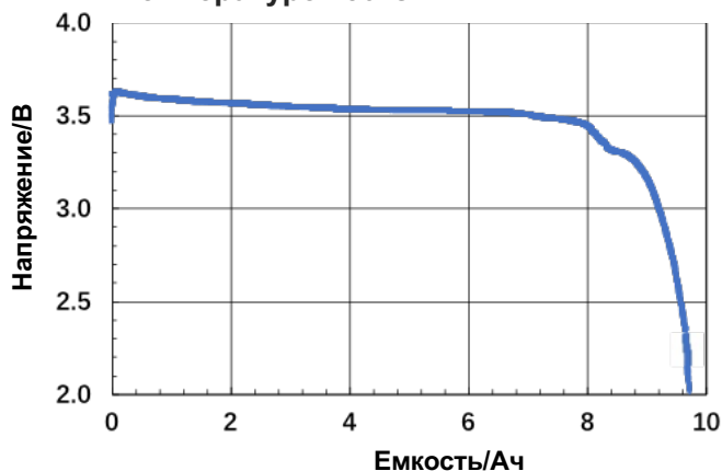
График разряда током 150 мА при температуре 150°C
