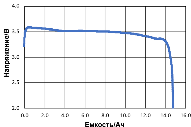
График разряда током 350 мА при температуре 100°C
