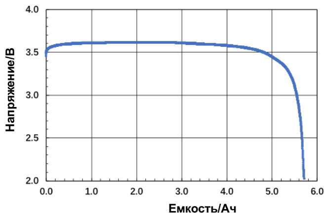
График разряда током 100 мА при температуре 80°C 100mA at 80°C
