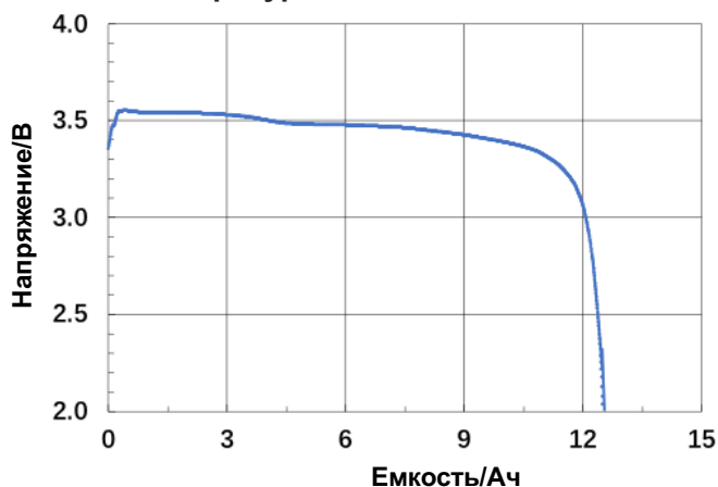
График разряда током 500 мА при температуре 150°C
